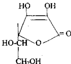
\gamma - Лактон-2,3-дегідро-L-гулонатної кислоти
